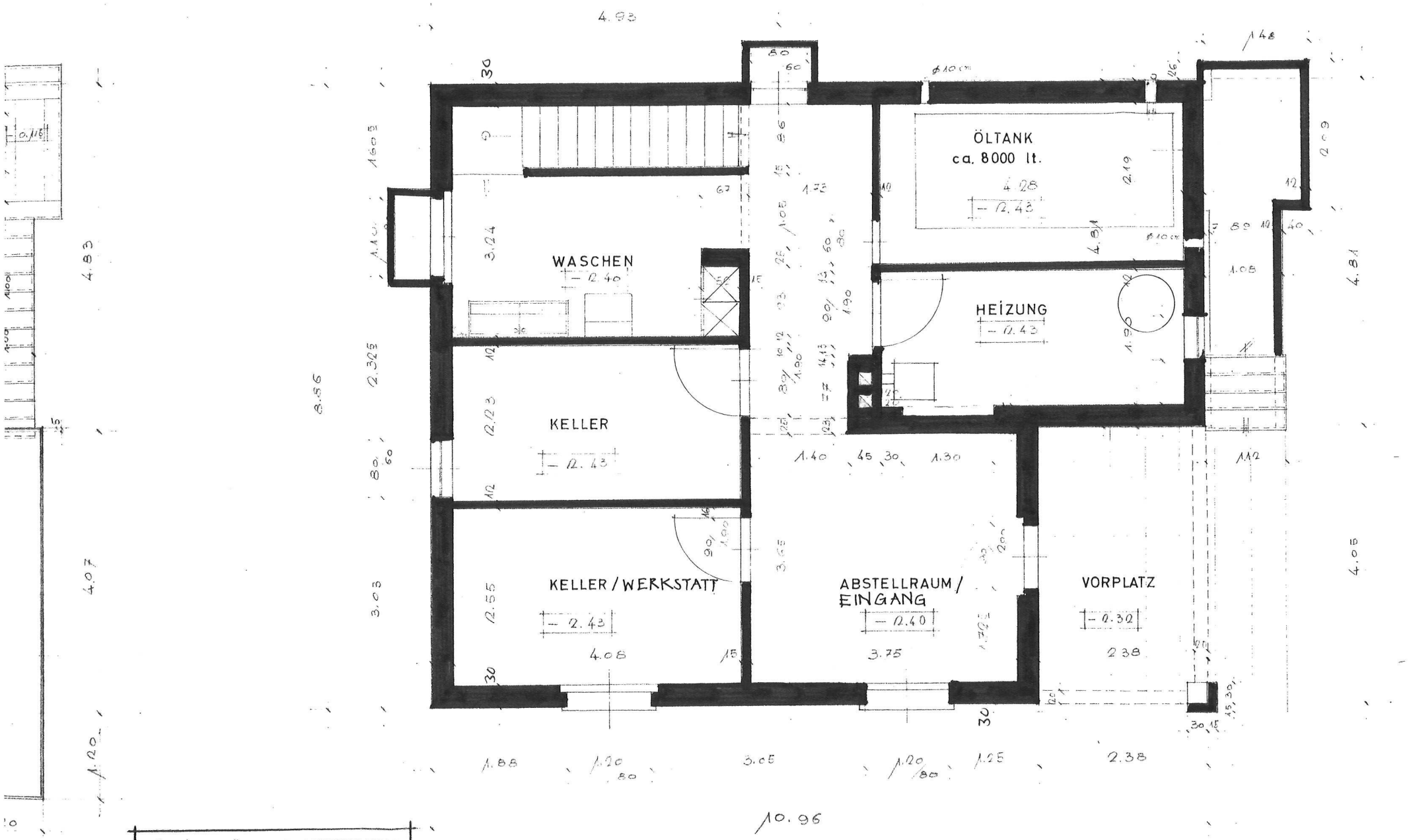
KELLER - GRUNDRISS.
